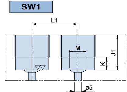
安裝底座示意圖 Mounting base diagram
